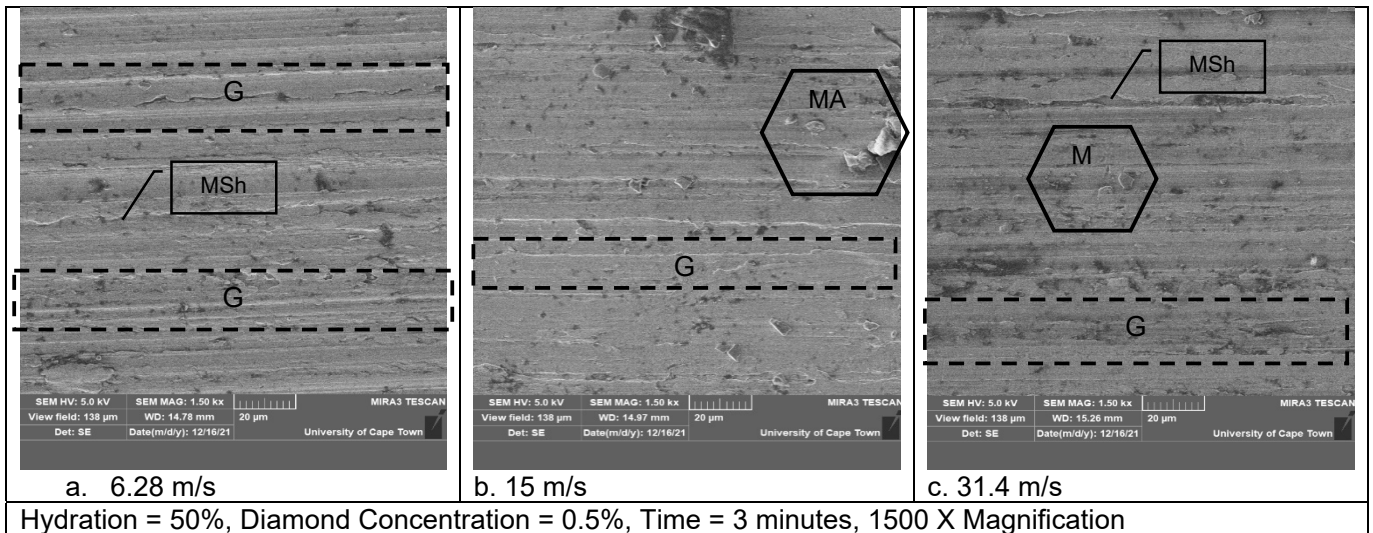
Figure 105 - 0.5%D, 3minutes, 50%H, 1500 X SEM Images
